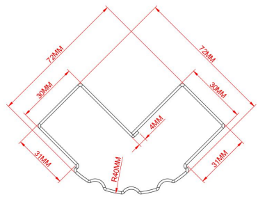
（边立柱截面线条示意图）
