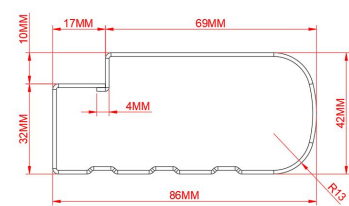
（横梁线条示意图）
