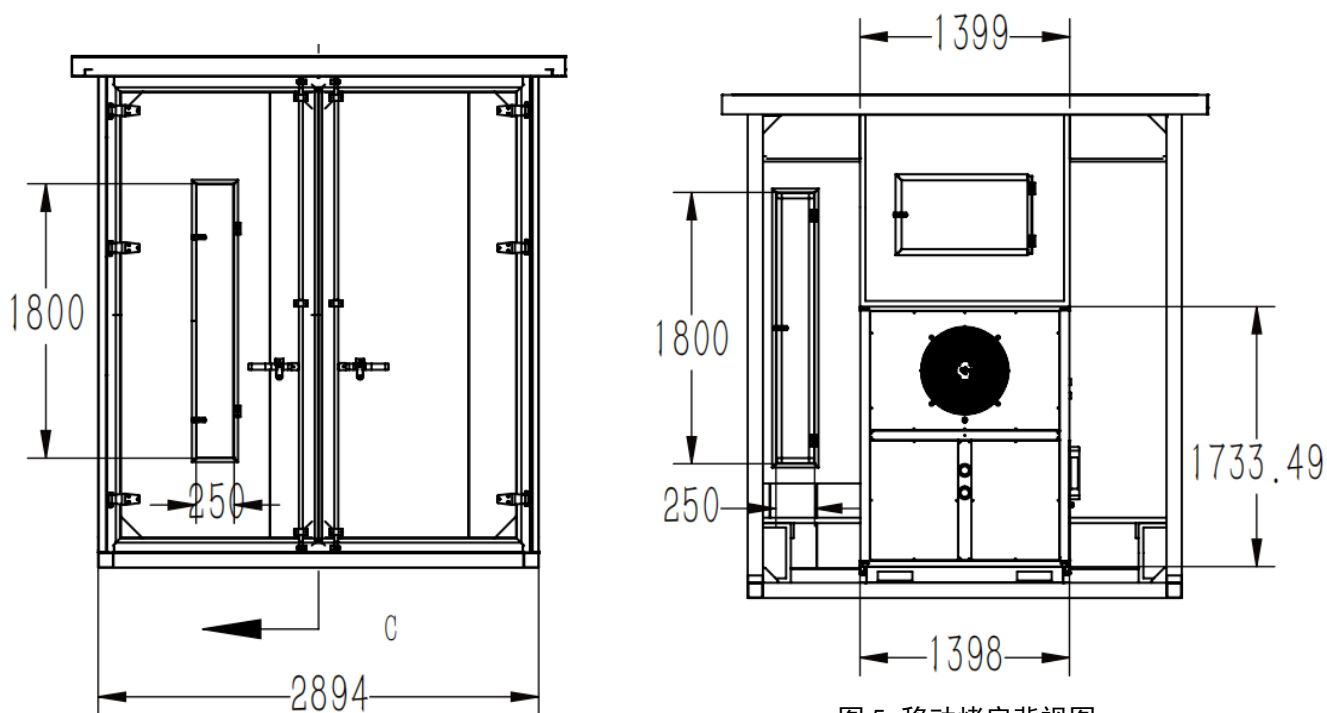
图 5 移动烤房背视图
